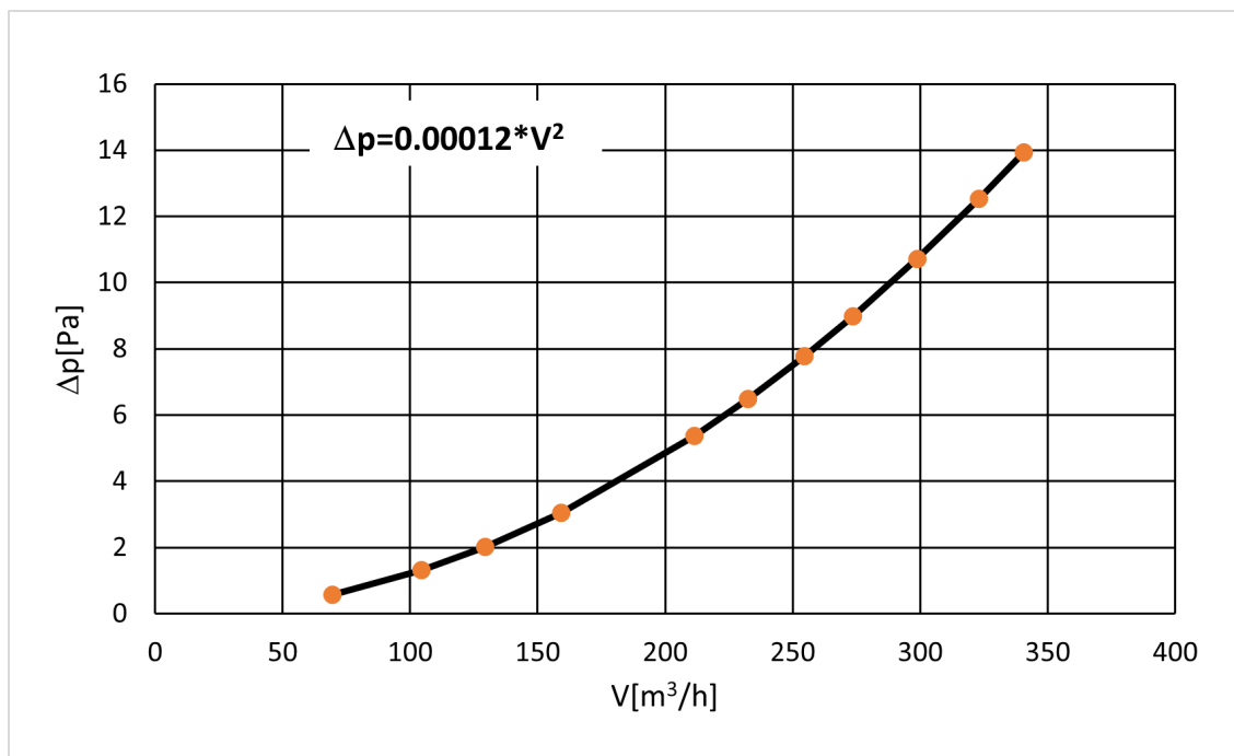
rys. 4. Charakterystyka hydrauliczna wyrzutni K2.
