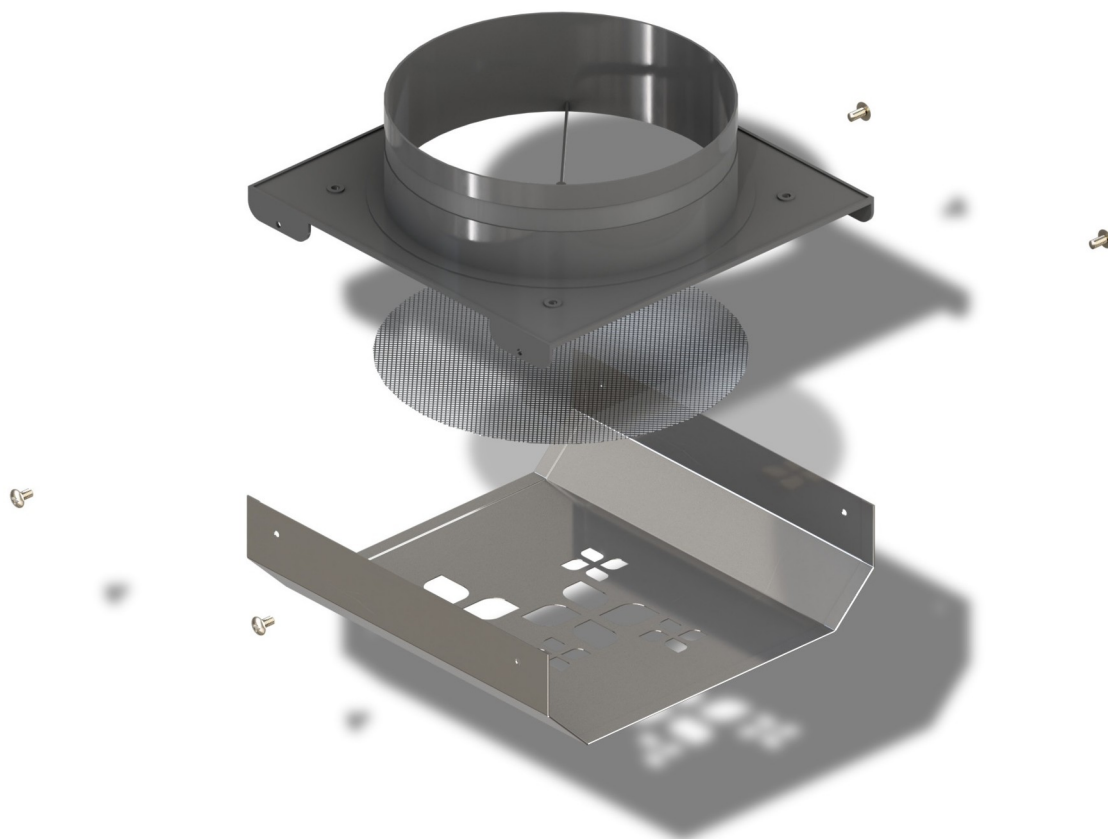
rys. 1. Rozstrzelony widok czerpni/wyrzutni K2.
