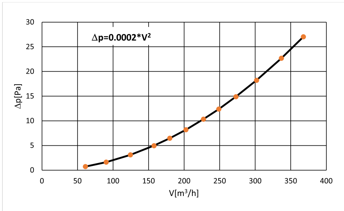
rys. 3. Charakterystyka hydrauliczna czepni K2.
