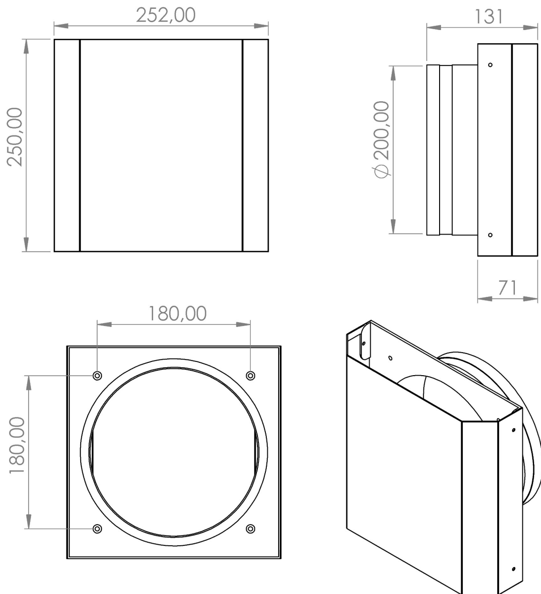
rys. 2. Wymiary czepni/wyrzutni K2.
