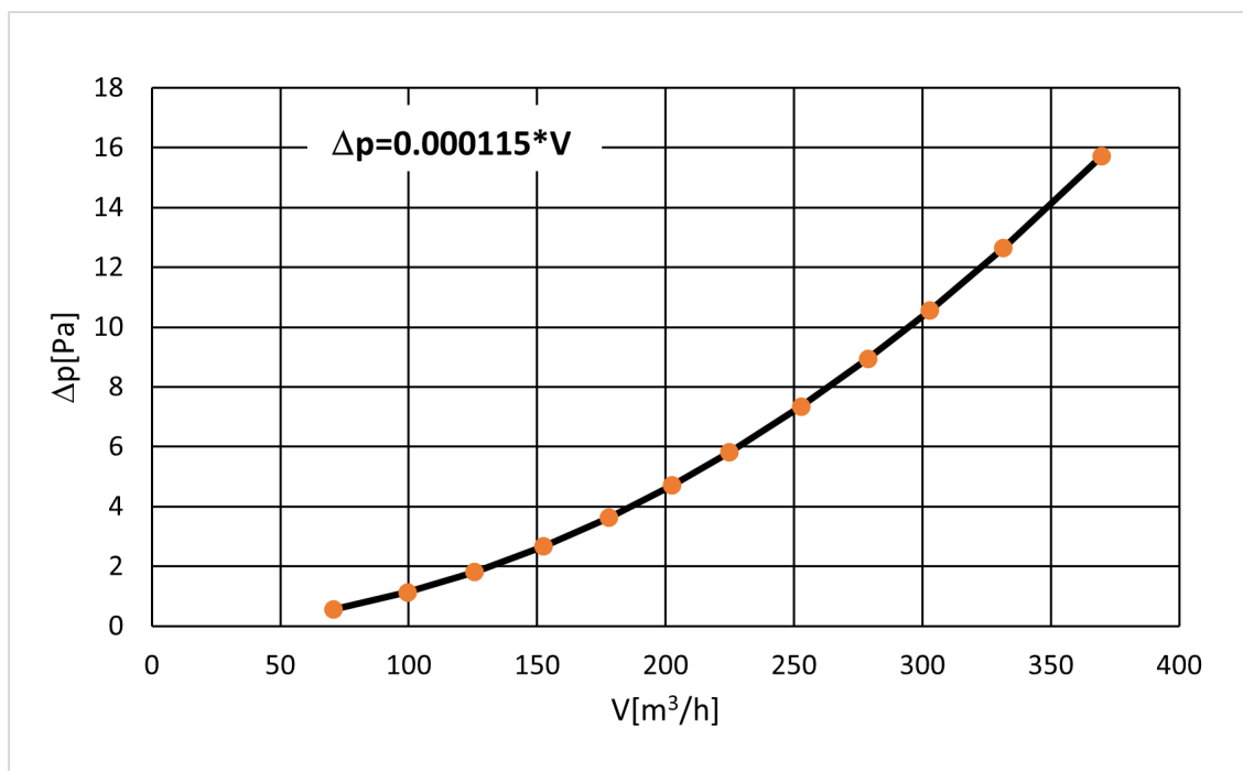
rys. 4. Charakterystyka hydrauliczna wyrzutni K4.
