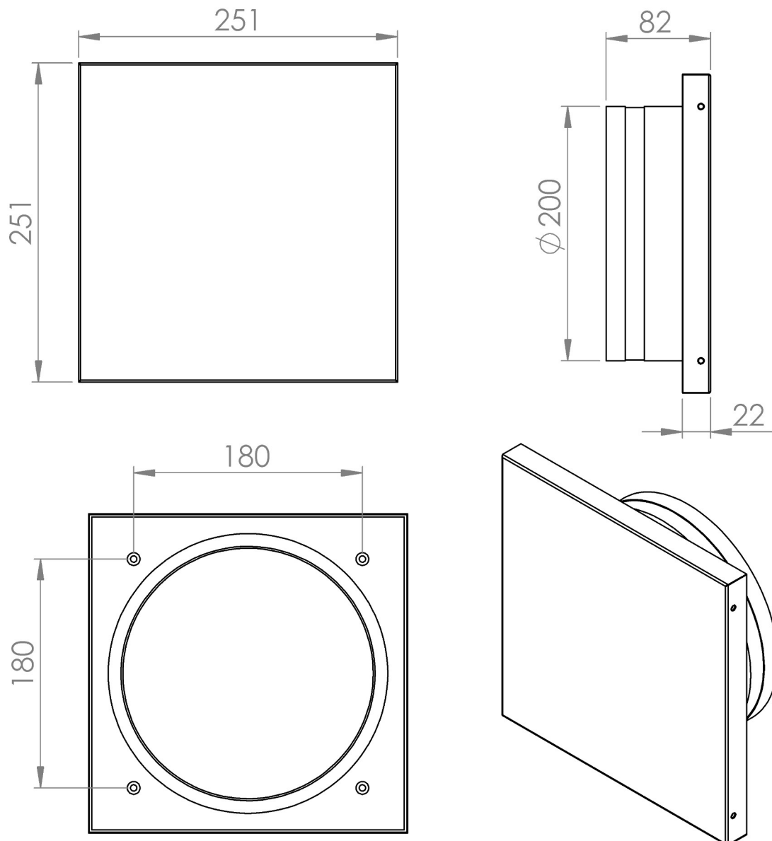
rys. 2. Wymiary czepni/wyrzutni K4.
