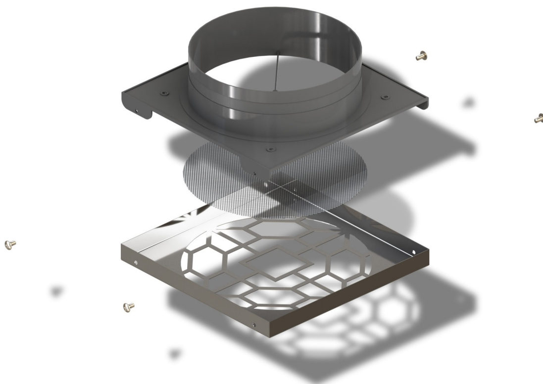
rys. 1. Rozstrzelony widok czerpni/wyrzutni K4.
