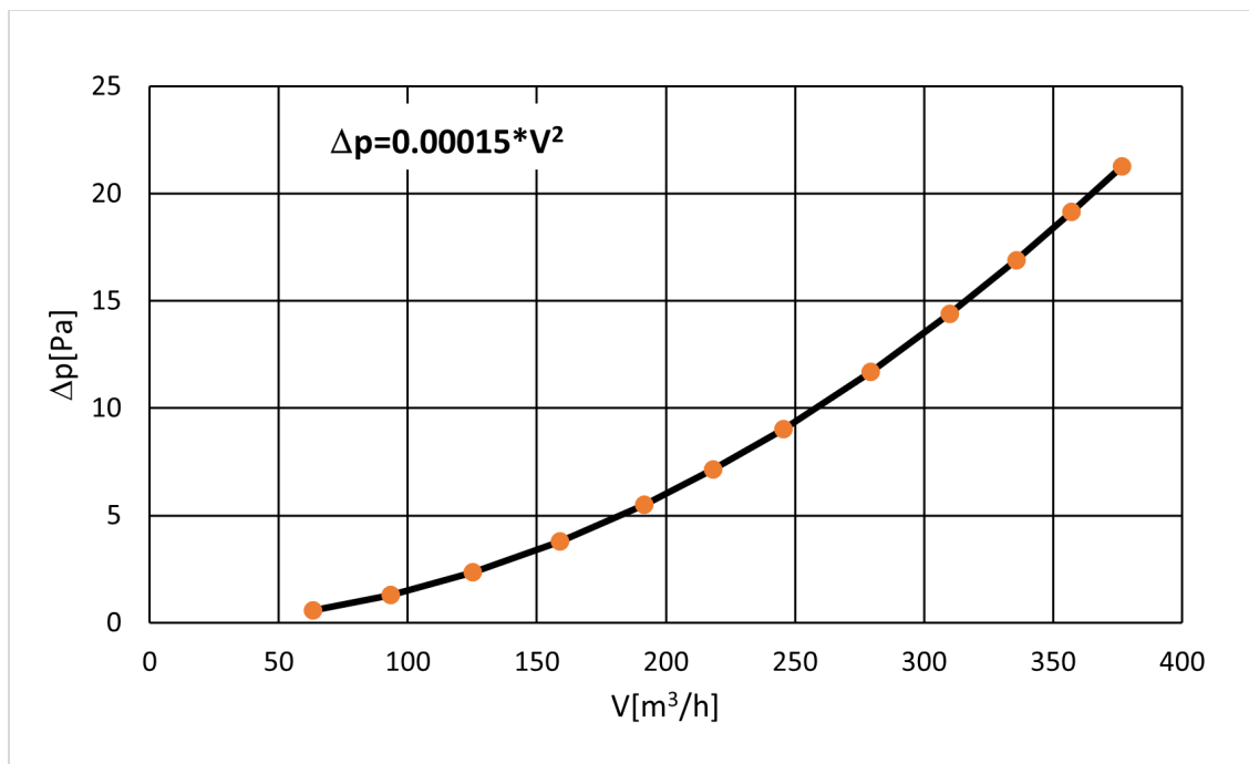
rys. 3. Charakterystyka hydrauliczna czepni K4.
