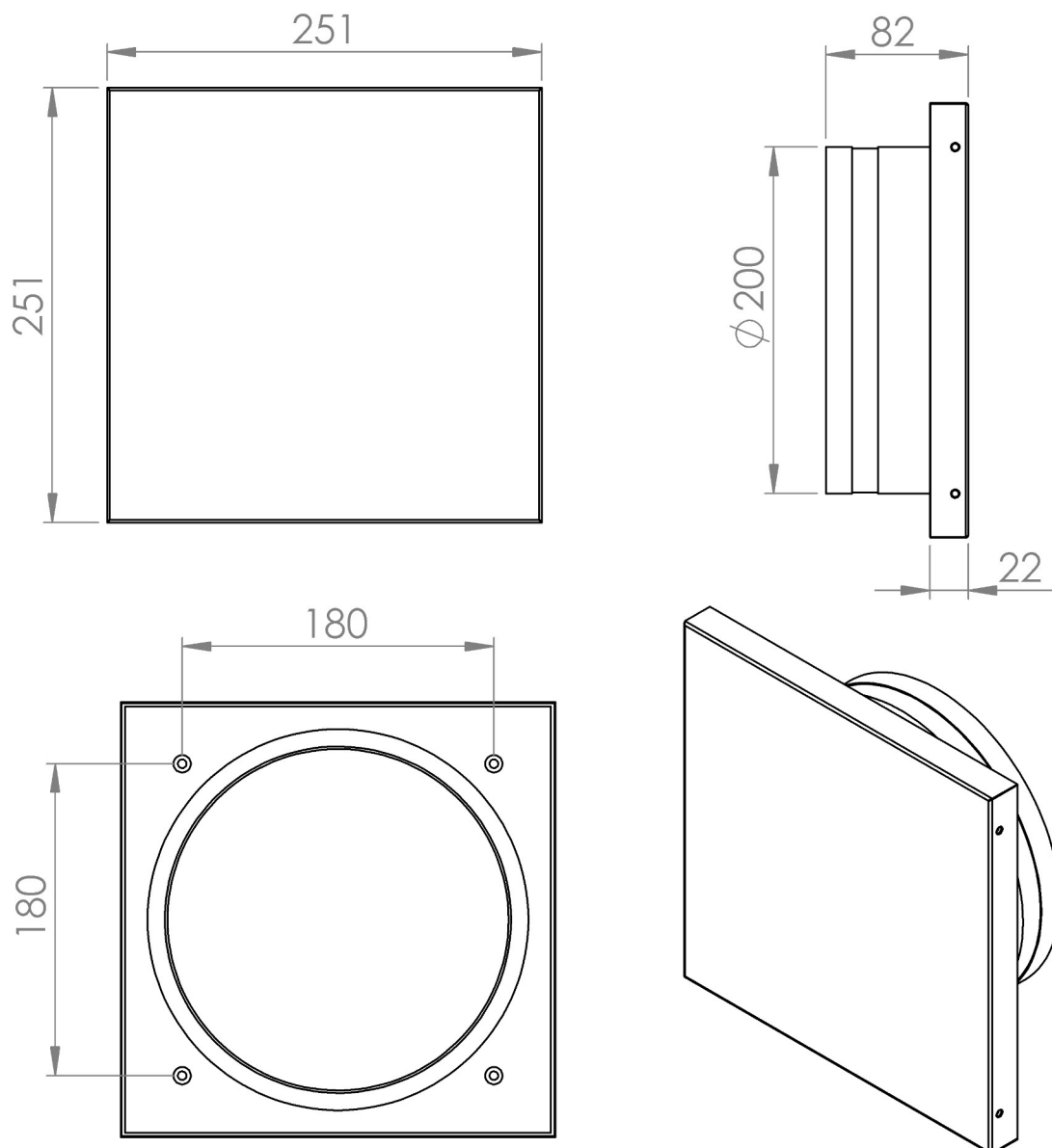
rys. 2. Wymiary czepni/wyrzutni K5.
