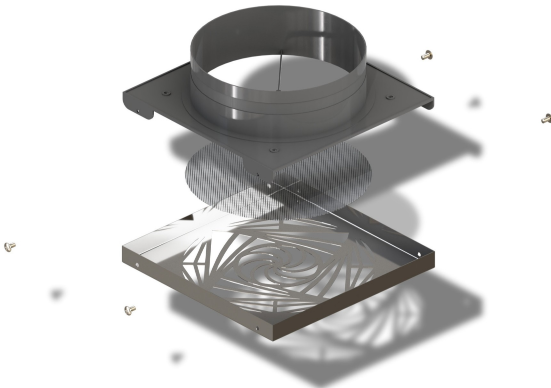
rys. 1. Rozstrzelony widok czerpni/wyrzutni K5.
