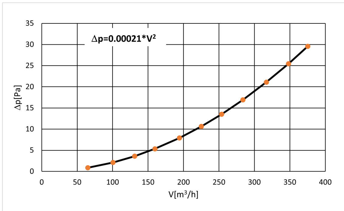
rys. 4. Charakterystyka hydrauliczna wyrzutni K5.
