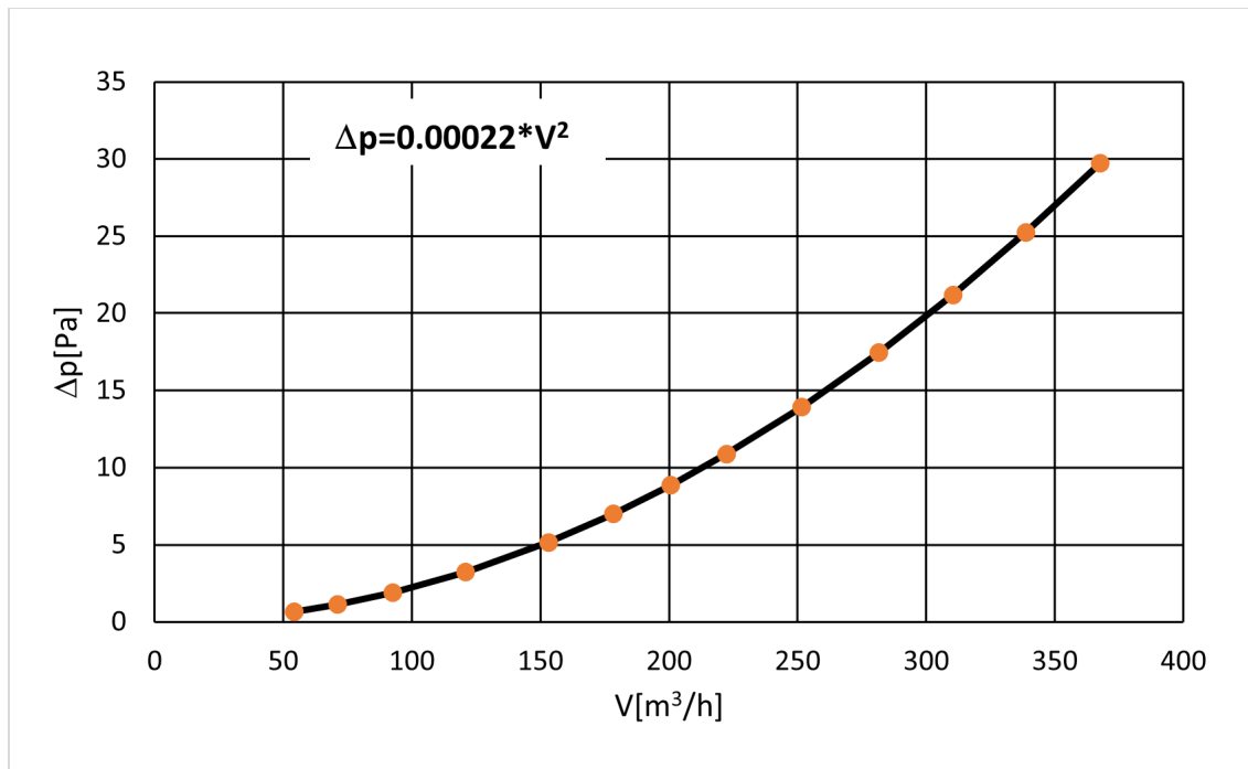
rys. 3. Charakterystyka hydrauliczna czepni K5.
