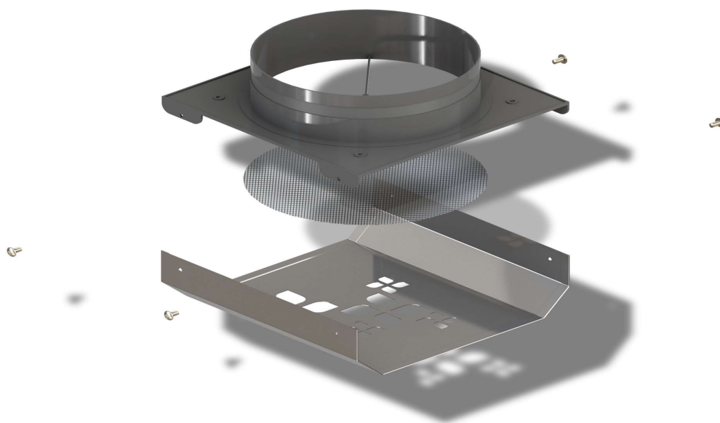
rys. 1. Rozstrzelony widok czerpni/wyrzutni K2-160.
