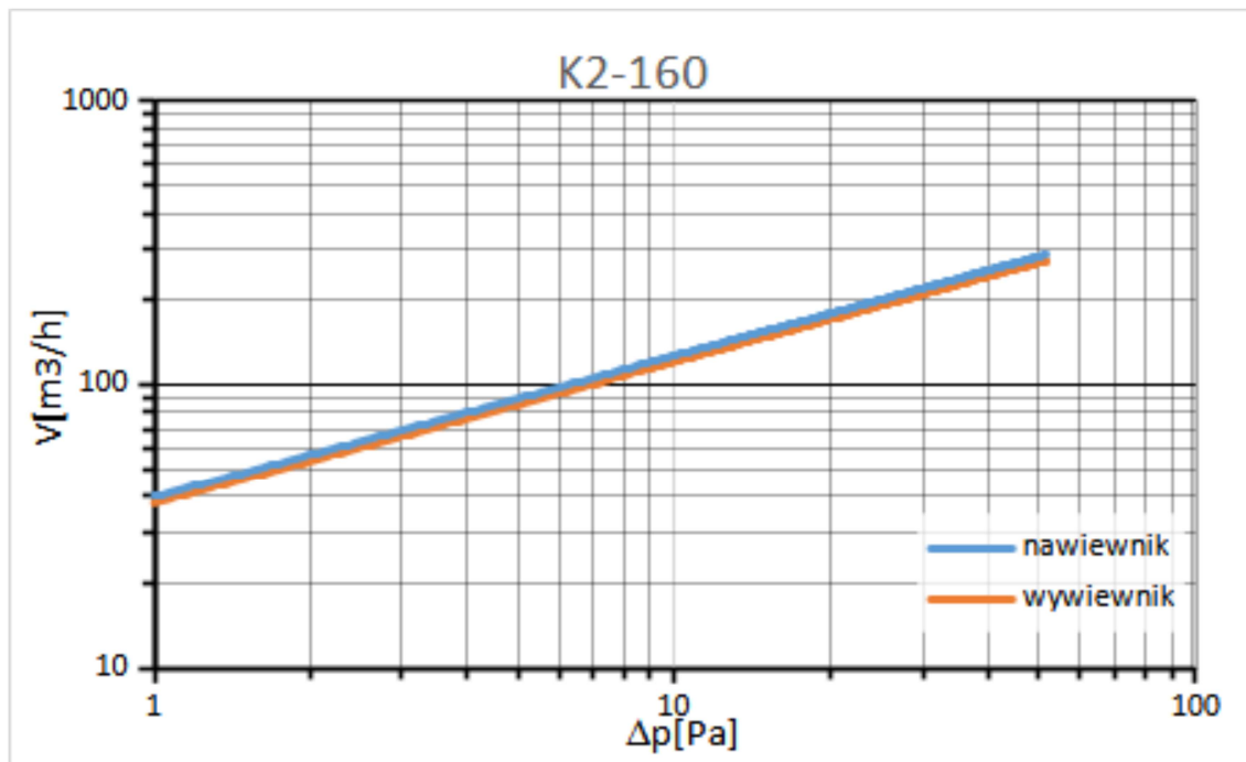
rys. 3. Charakterystyka hydrauliczna czepni K2-160.
