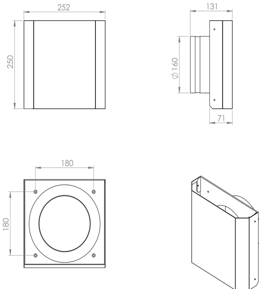
rys. 2. Wymiary czepni/wyrzutni K2-160.
