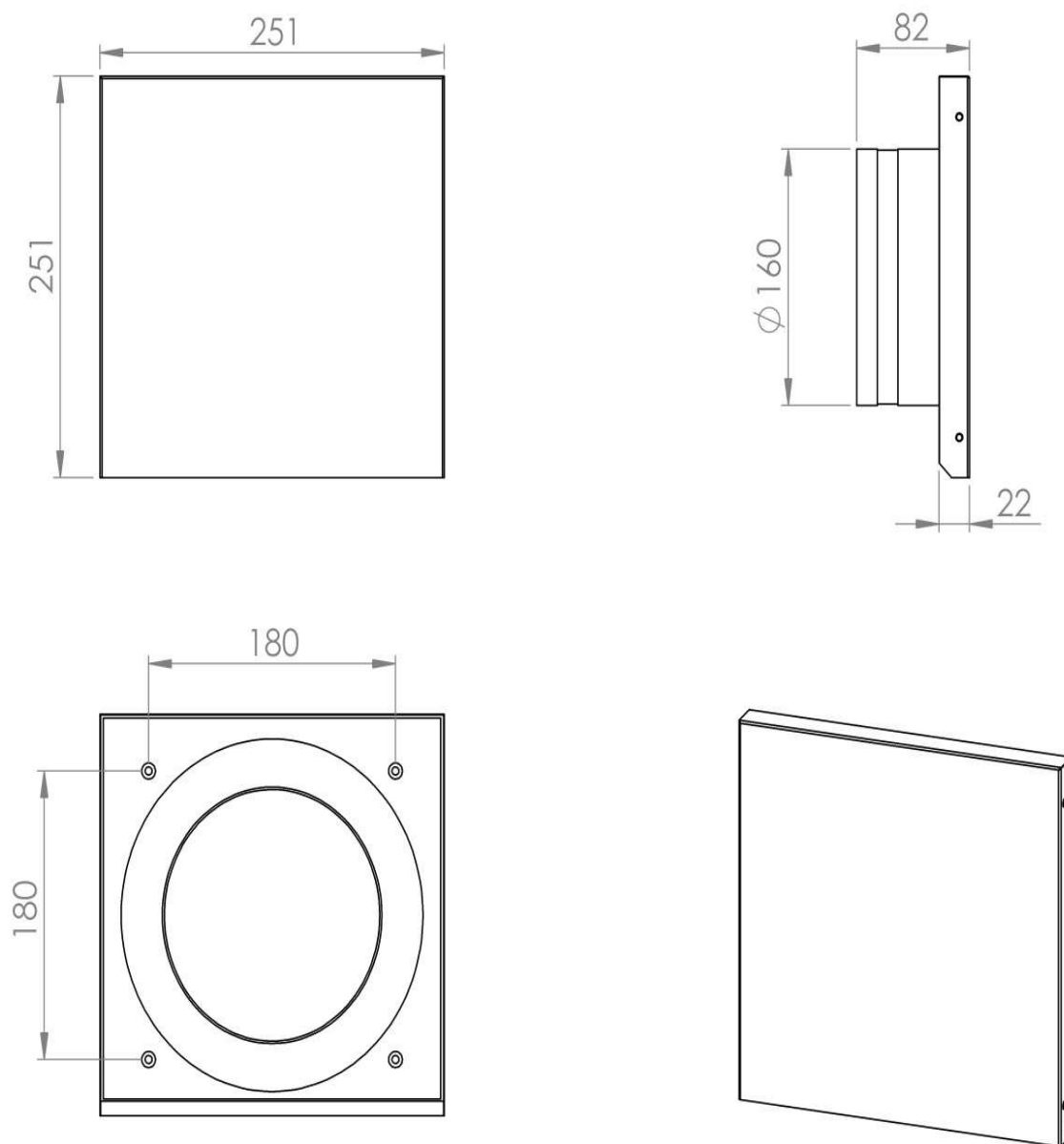
rys. 2. Wymiary czepni/wyrzutni K5-160.
