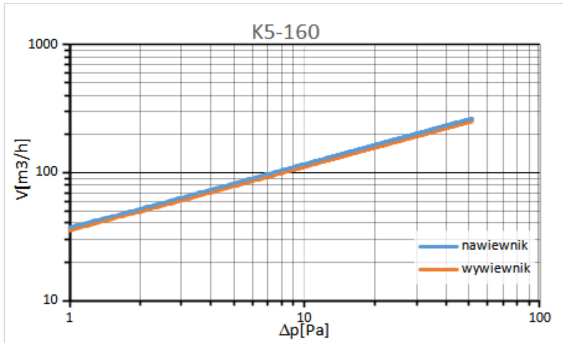
rys. 3. Charakterystyka hydrauliczna czepni K5-160.
