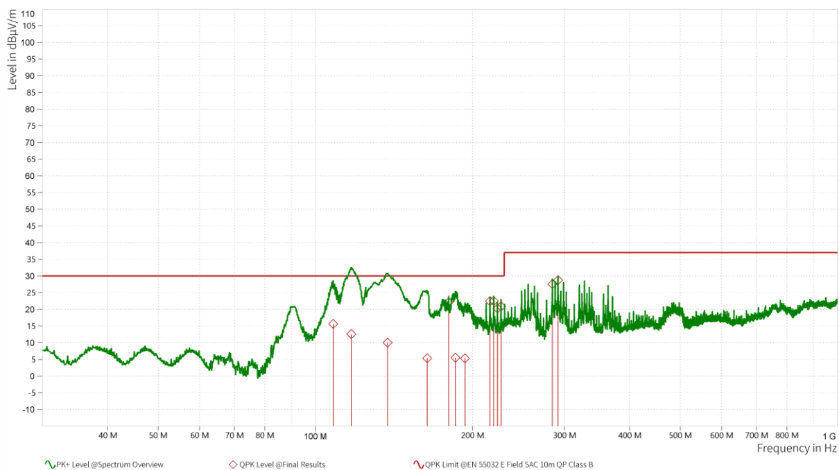
Rys. 8.8.1 Wyniki pomiaru poziomu emisji zaburzeń elektromagnetycznych promieniowanych w zakresie częstotliwości 30 MHz ÷ 1GHz, polaryzacja pionowa
