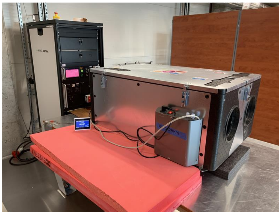
Fot. 8.4.1 Stanowisko badań
