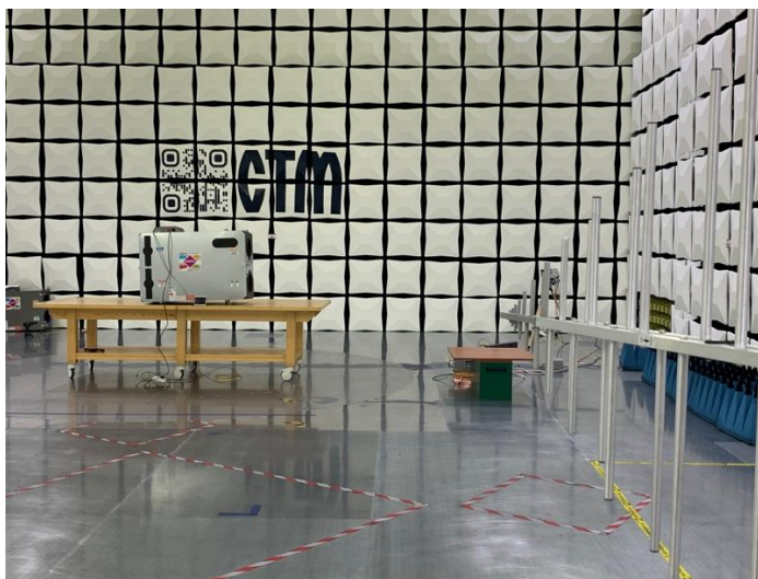
Fot. 8.8.1 Stanowisko badań
