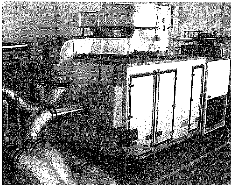
Rys. 1. Widok ogólny stanowiska do badań central wentylacyjnych
