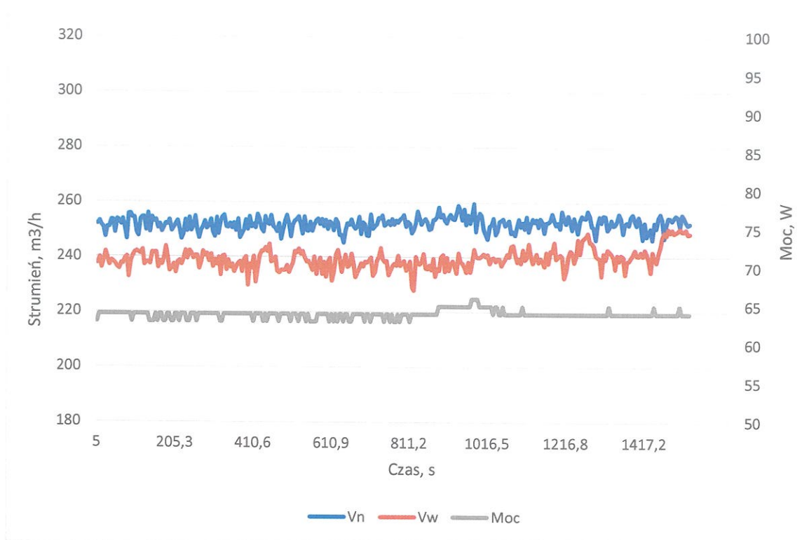
Wyk.3. Przebieg zmian strumieni powietrza oraz mocy dla serii pomiarowej nr 1.
