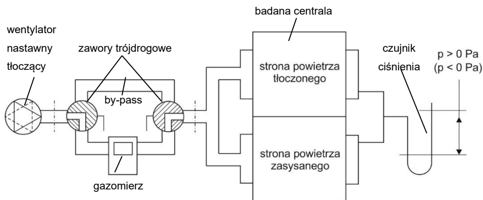
Rys. 2. Schemat układu do badania szczelności zewnętrznej central wentylacyjnych z odzyskiem ciepła
