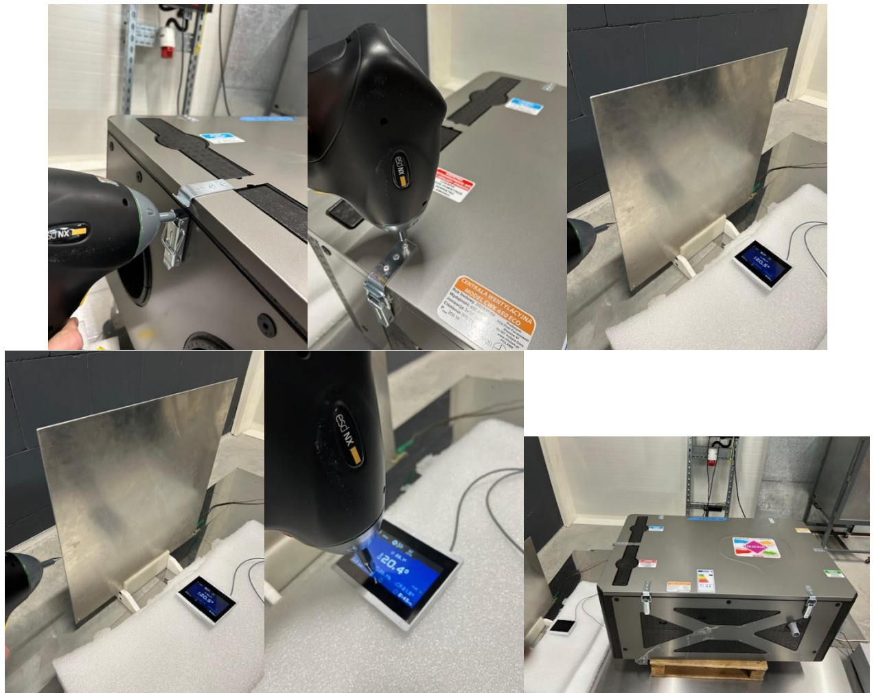
Fot. 8.1.1 Stanowisko badań
