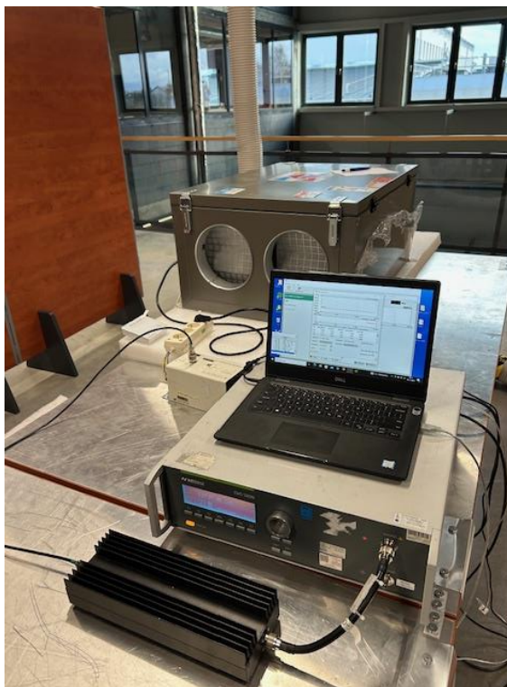
Fot. 8.5.1 Stanowisko badań
