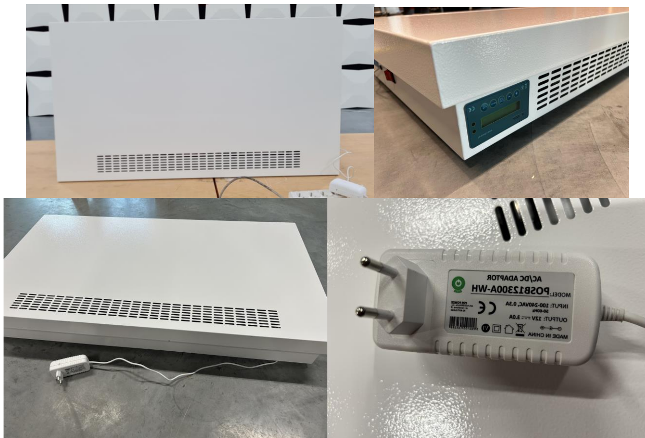
Fot. 3.5.1 Obiekt badań
