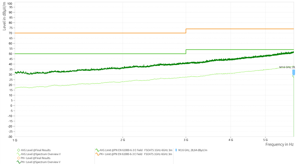
Rys. 8.7.2 Wyniki pomiaru poziomu emisji zaburzeń elektromagnetycznych promieniowanych w zakresie częstotliwości 30 MHz ÷ 1GHz, polaryzacja pozioma.
