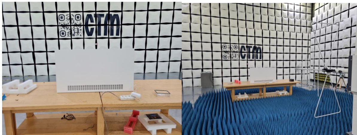
Fot. 8.7.1 Stanowisko badań
