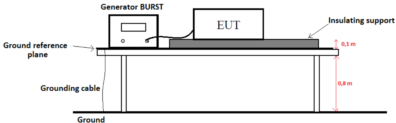
Rys. 8.2.1 Schemat blokowy stanowiska do badań odporności na serie szybkich elektrycznych stanów przejściowych (BURST)
