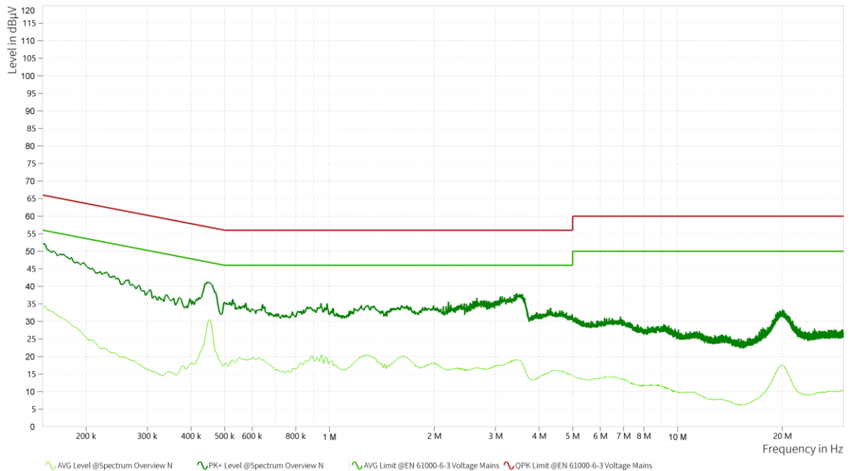
Rys. 8.6.2 Pomiar poziomu emisji przewodzonych w zakresie częstotliwości 150kHz ÷ 30MHz, linia N
