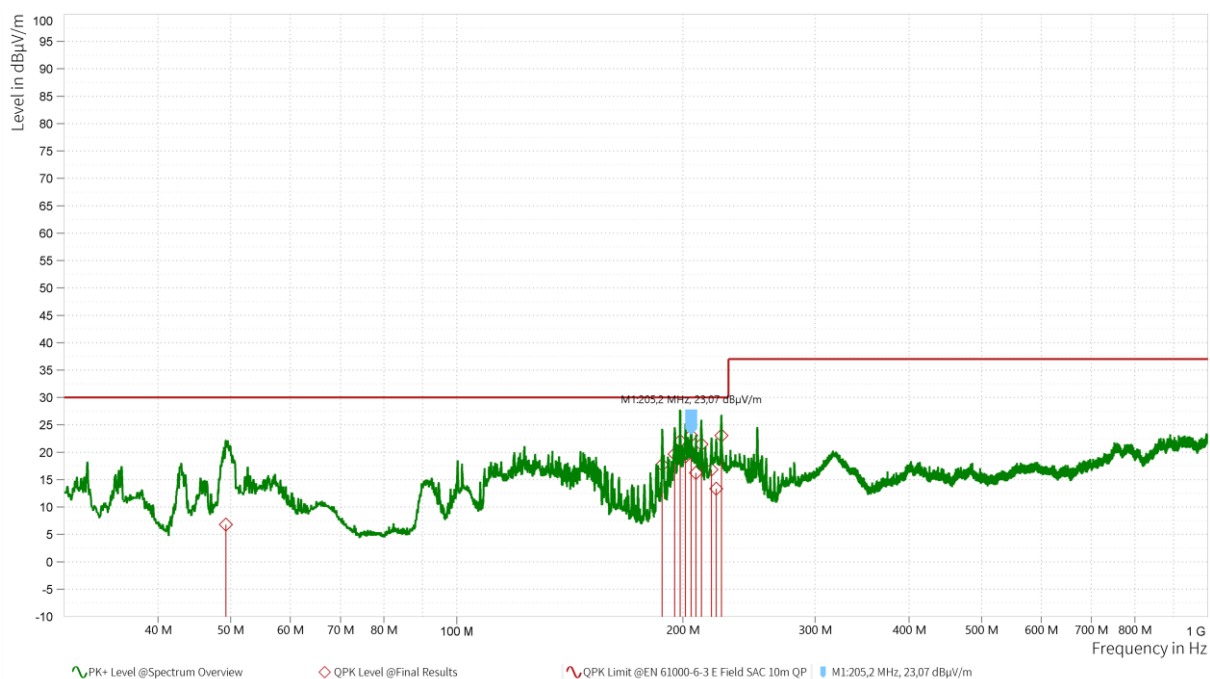
Rys. 8.7.1 Wyniki pomiaru poziomu emisji zaburzeń elektromagnetycznych promieniowanych w zakresie częstotliwości 30 MHz ÷ 1GHz, polaryzacja pionowa
