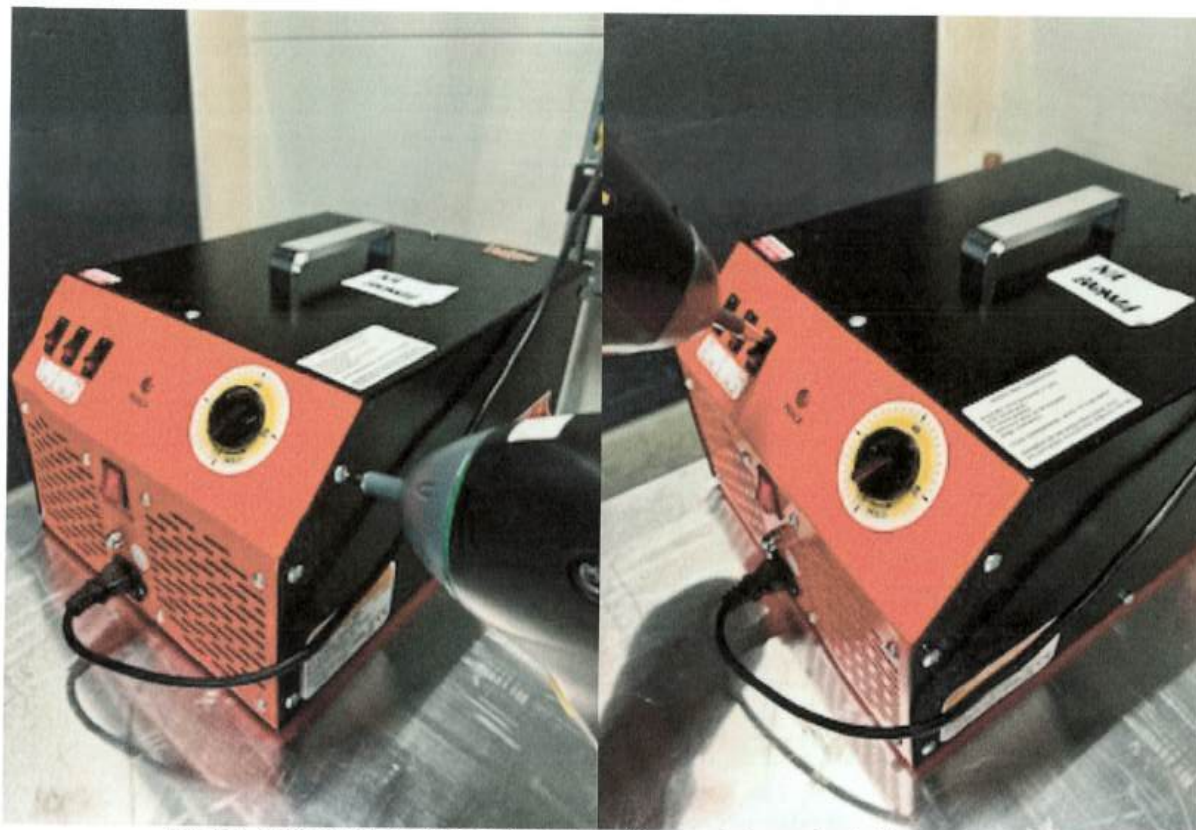
Fot. 8.1.1 Stanowisko do badań odporność na wyładowania elektrostatyczne
