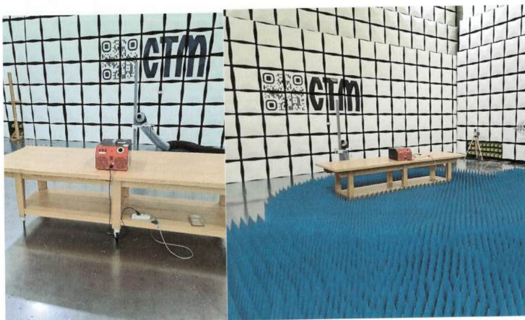
Fot. 8.8.1 Stanowisko do badań
