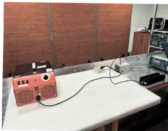
Fot. 8.5.1 Stanowisko do badań
