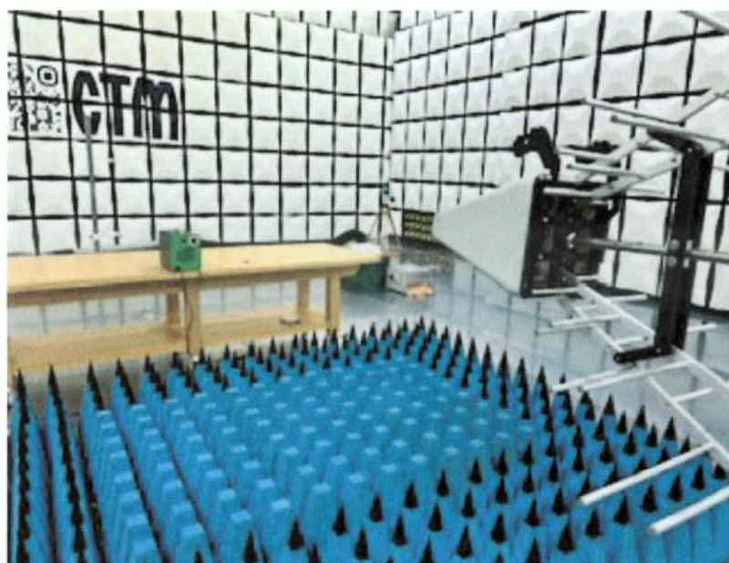
Fot. 8.2.1 Stanowisko do badań odporności na pole elektromagnetyczne (80MHz ÷ 6GHz)
