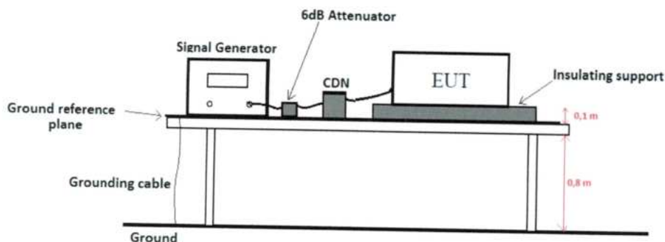
Rys. 8.5.1 Schemat blokowy stanowiska odporności na zakłócenia przewodzone w zakresie częstotliwości od 150 kHz do 80MHz
