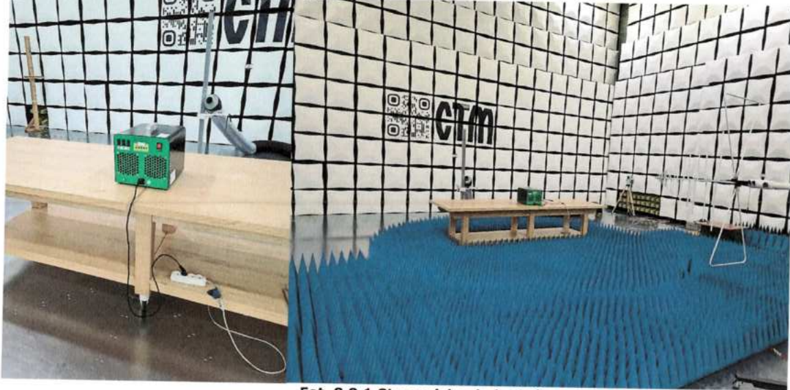
Fot. 8.8.1 Stanowisko do badań
