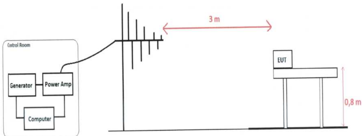
Rys. 8.2.1 Schemat blokowy stanowiska do badań
