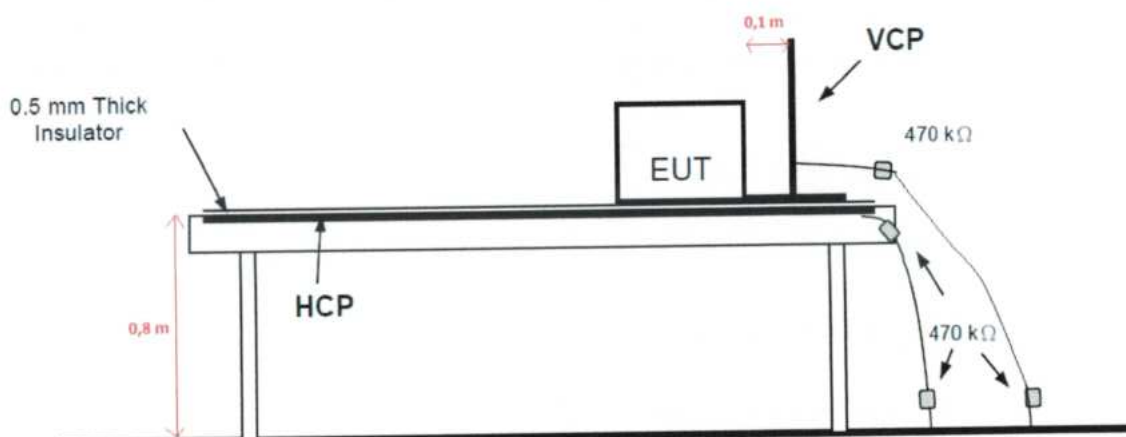
Rys. 8.1.1 Schemat blokowy stanowiska do badań odporność na wyładowania elektrostatyczne
