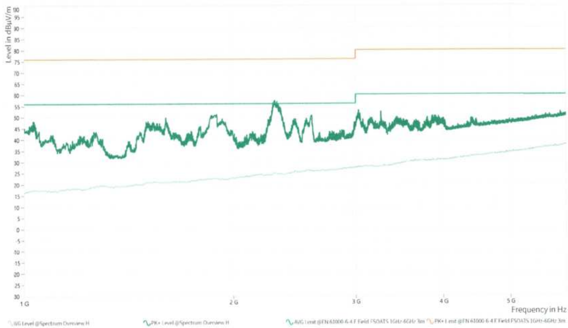
Rys. 8.8.3 Wyniki pomiaru poziomu emisji zaburzeń elektromagnetycznych promieniowanych w zakresie częstotliwości 1 GHz ÷ 6GHz, polaryzacja pozioma
