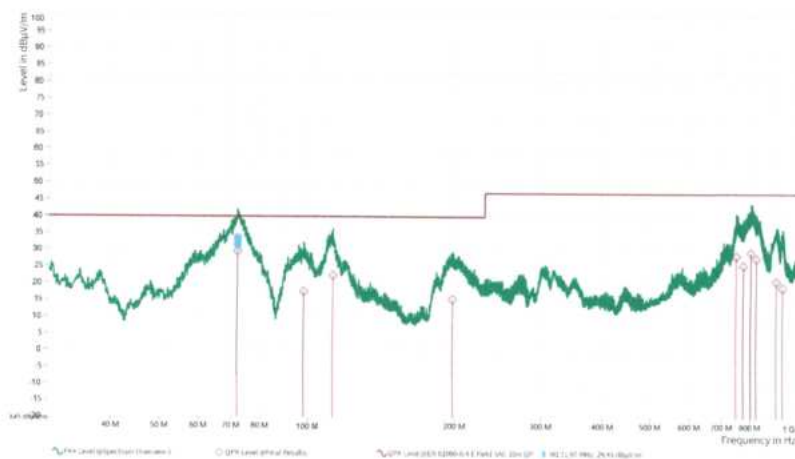
Rys. 8.8.1 Wyniki pomiaru poziomu emisji zaburzeń elektromagnetycznych promieniowanych w zakresie częstotliwości 30 MHz ÷ 1GHz, polaryzacja pozioma
