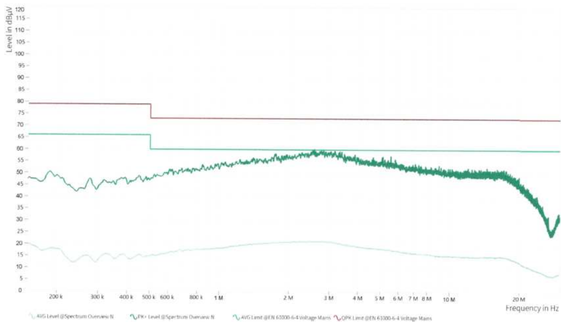
Rys.8.7.1 Pomiar poziomu emisji przewodzonych w zakresie częstotliwości 150kHz ÷ 30MHz, linia L
