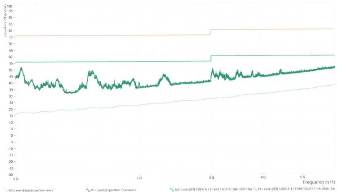
Rys.8.8.4 Wyniki pomiaru poziomu emisji zaburzeń elektromagnetycznych promieniowanych w zakresie częstotliwości 1 GHz ÷ 6 GHz, polaryzacja pionowa
