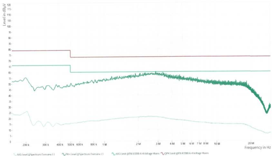
Rys.8.7.2 . Pomiar poziomu emisji przewodzonych w zakresie częstotliwości 150kHz ÷ 30MHz, linia N
