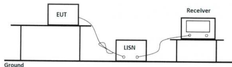
Rys.8.7.1. Schemat stanowiska do pomiaru poziomu emisji zaburzeń elektromagnetycznych przewodzonych
