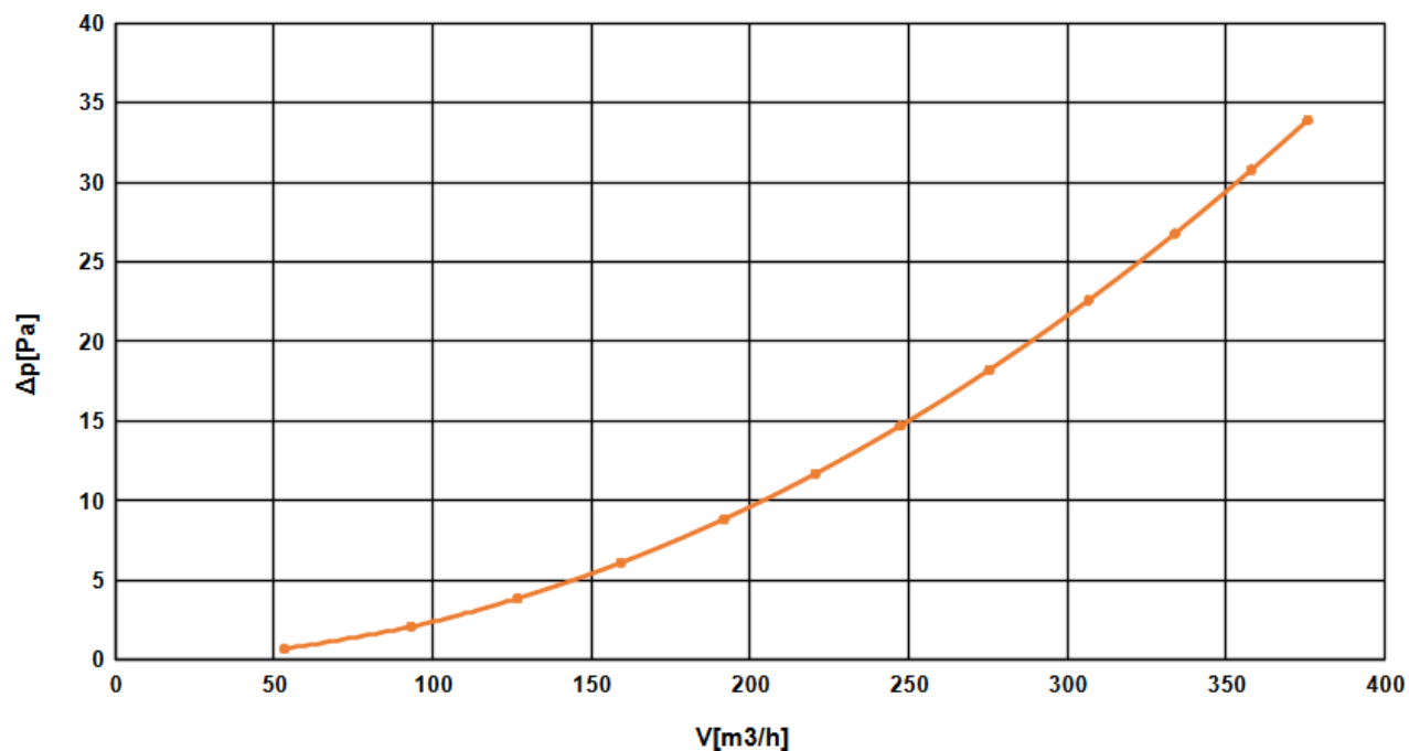
Rysunek 3: Charakterystyka hydrauliczna czerpni CWK2.
