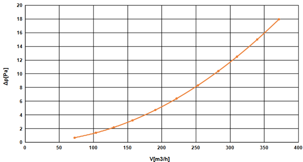
Rysunek 4: Charakterystyka hydrauliczna wyrzutni CWK2.
