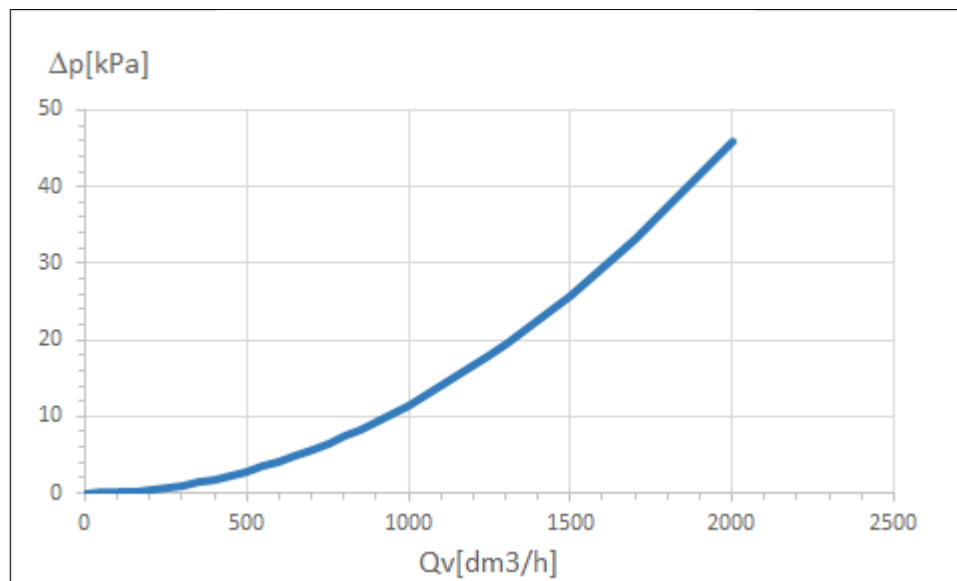
rys. 3. Charakterystyka oporów hydraulicznych nagrzewnicy po stronie wody.
