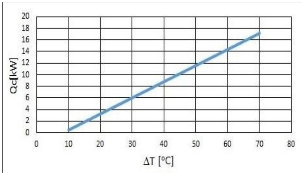
rys. 1. Charakterystyka mocy nagrzewnicy w średniej różnicy funkcji \Delta T .
