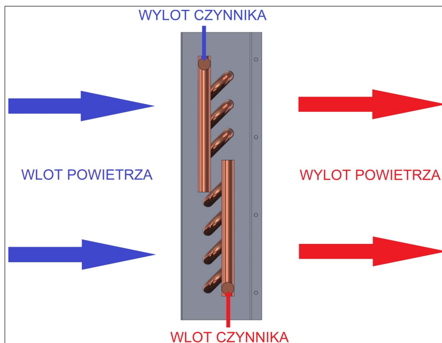
rys. 5. Schemat podłączenia wymiennika względem przepływającego powietrza.
