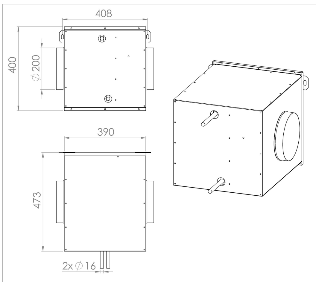
rys.4. Wymiary nagrzewnicy.
