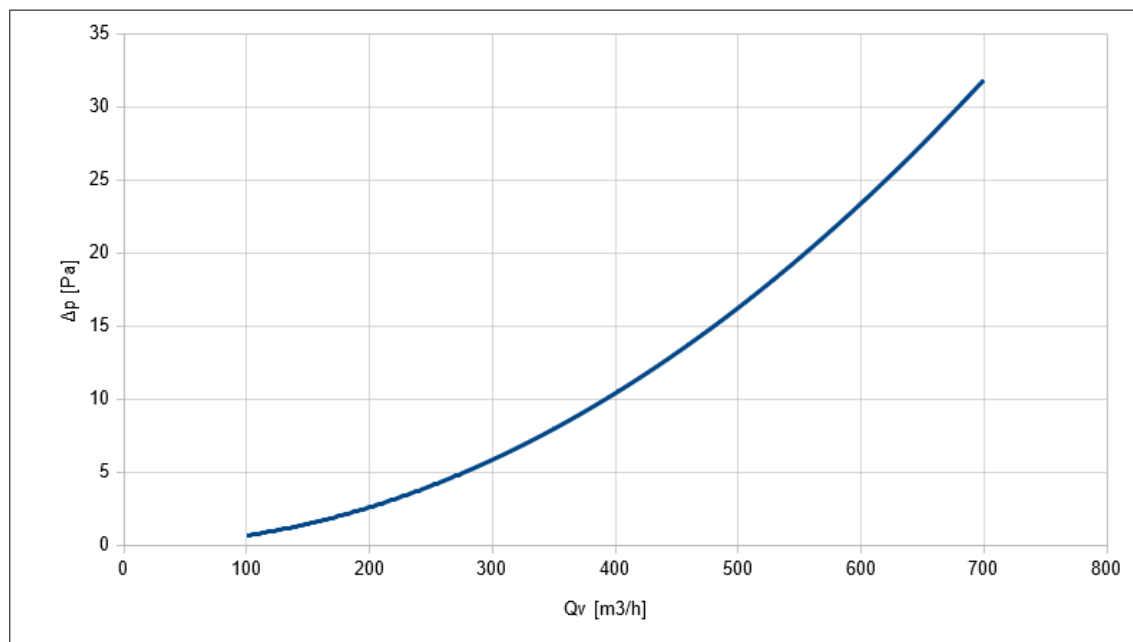
rys. 2. Charakterystyka oporów hydraulicznych nagrzewnicy po stronie powietrza.
